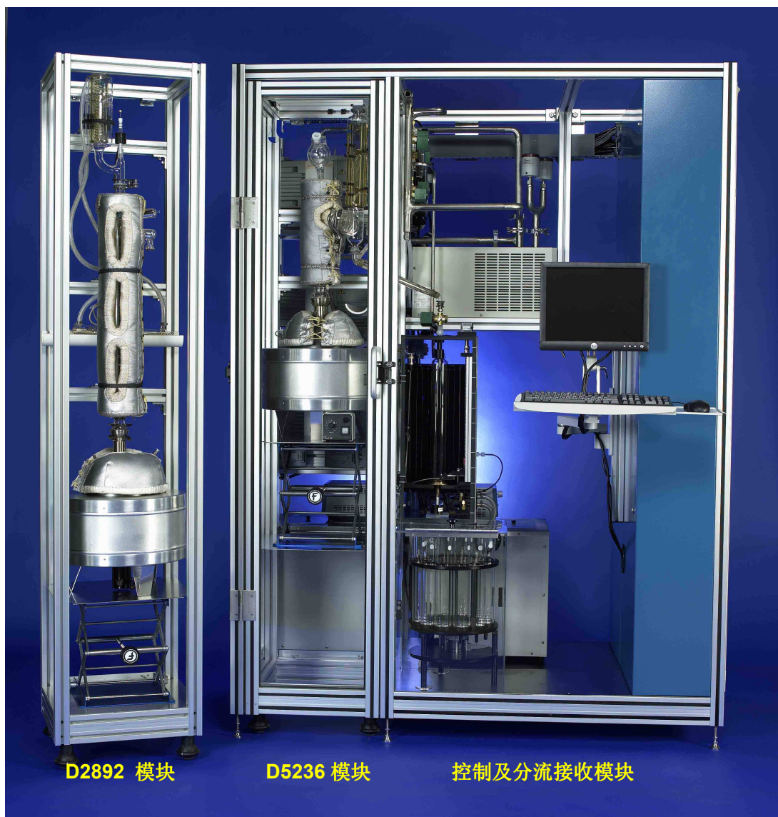
图三：AUTOMAXX 9100 全自动实沸点原油蒸馏系统
